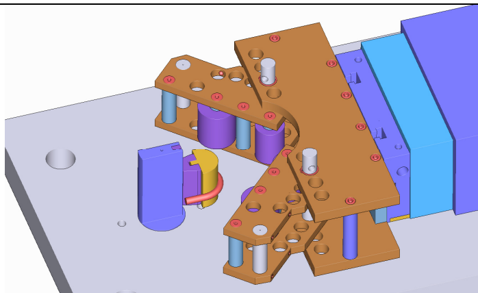
Špeciálny prípravok na ohyb 180° Special tooling for 180 degrees bendings
