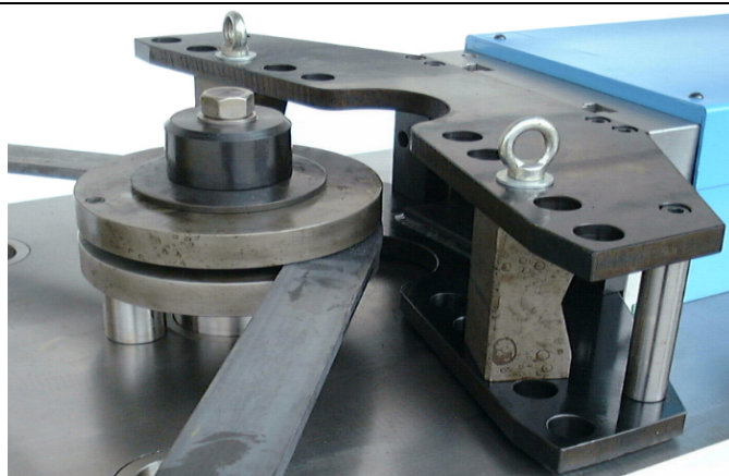
Prípravok na ohýbanie plochej ocele do max. bending on edge up to 50 x 8 mm
