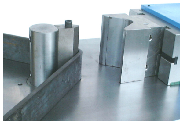
Prípravok na ohýbanie rúr do pipe bending up to 48 mm, max. 90°
