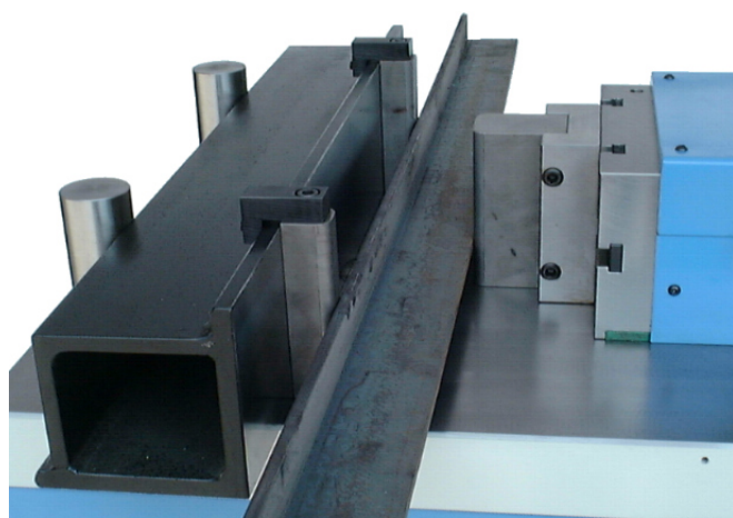
Vyrovnávací prípravok nosičov do výšky straightening of H-beam , T-profile and other profiles up to 140 mm
