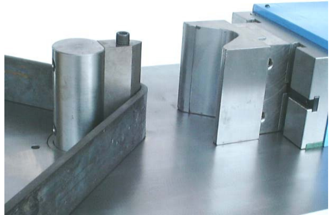
Biegewerkzeug für Rohre bis pipe bending up to 60 mm, max. 90°
